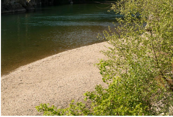
Banc de galets en rive gauche en amont du Pont du Gard.
