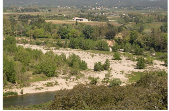
Banc de galets en cours de végétalisation dans le méandre amont de Saint-Privat.
